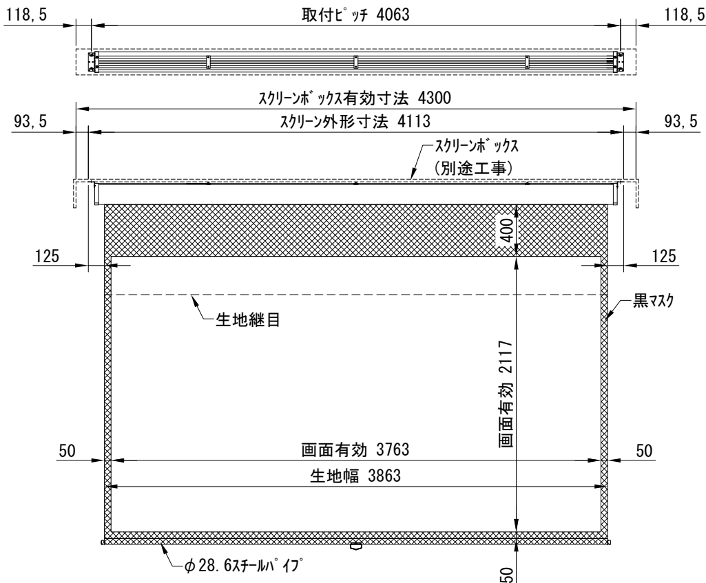
外観図 1/40
