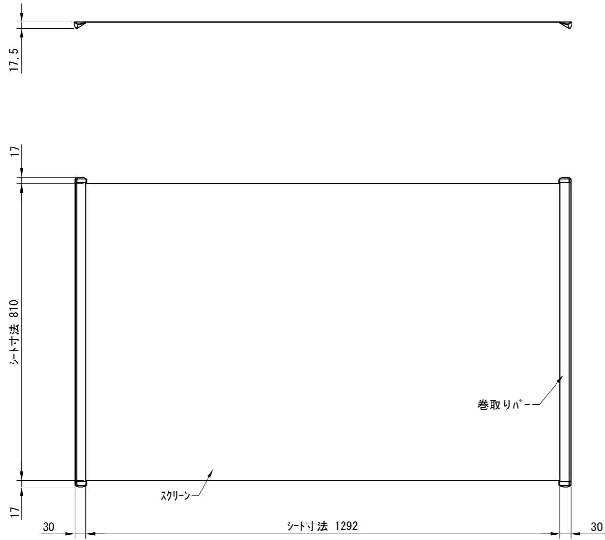
外観図 1/30
