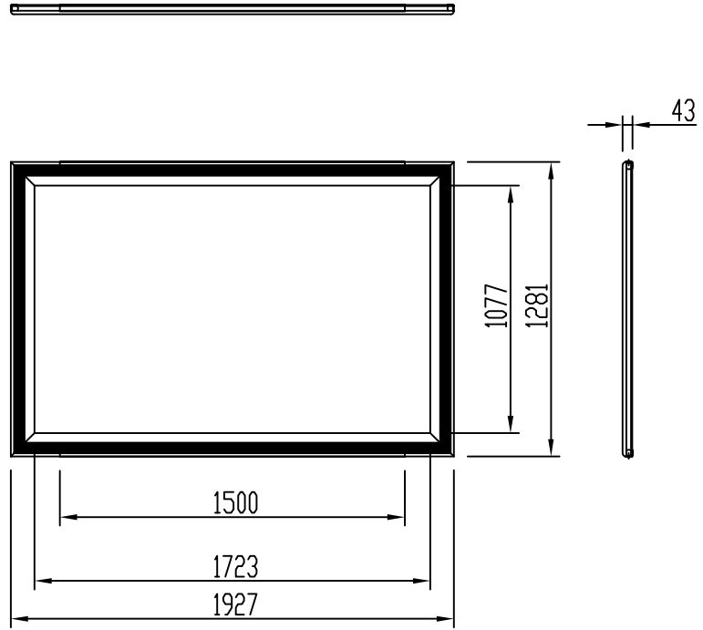
外観図 1/40
