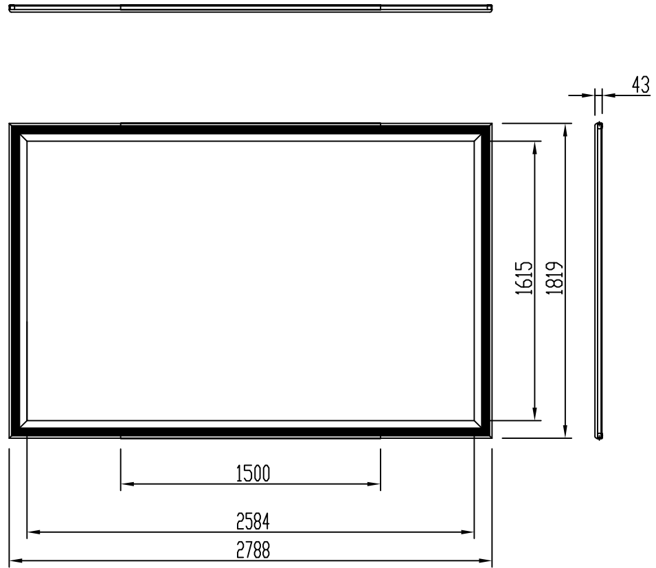
外観図 1/40
