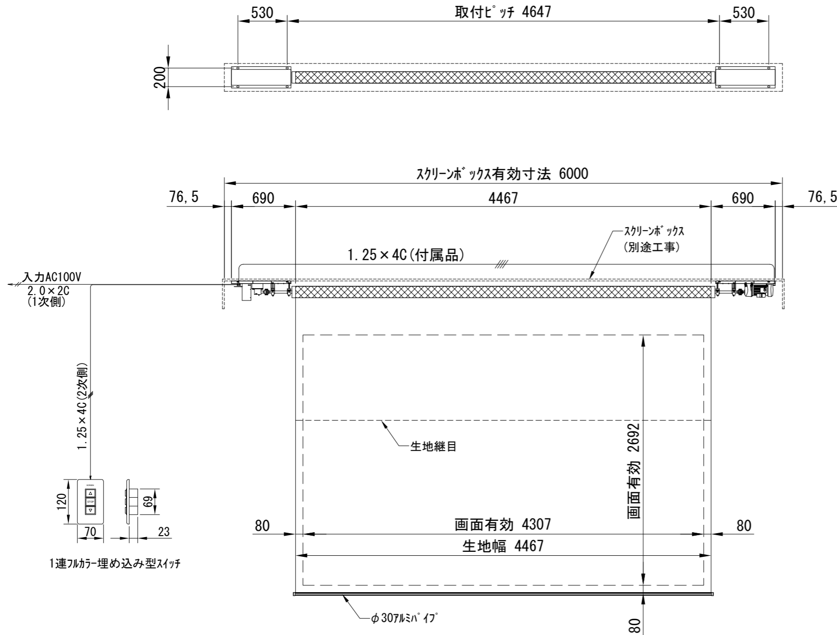
外観図 1/40
