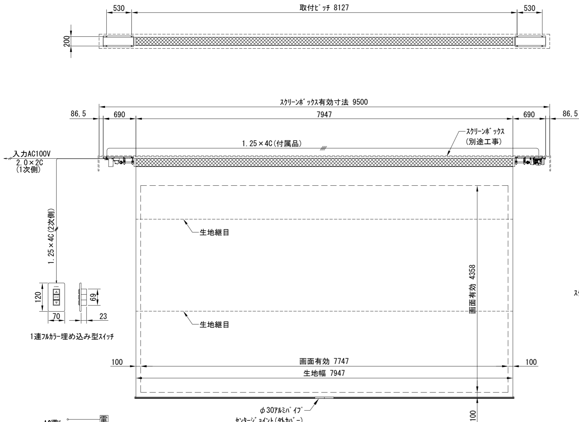
外観図 1/50
