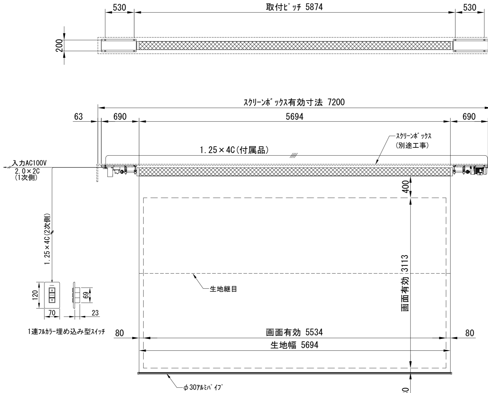
外観図 1/40
