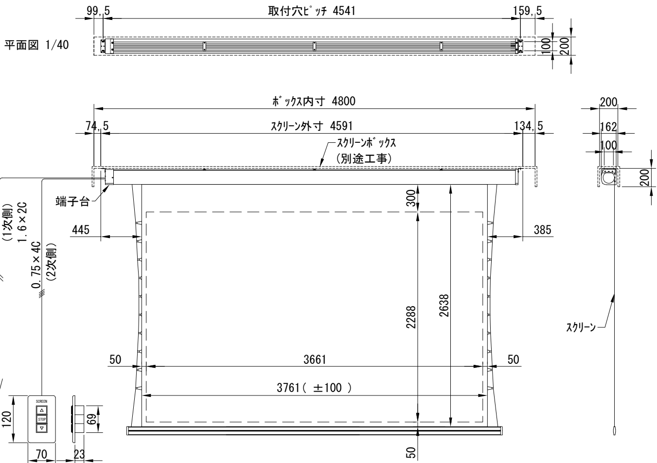
外観図 1/40
